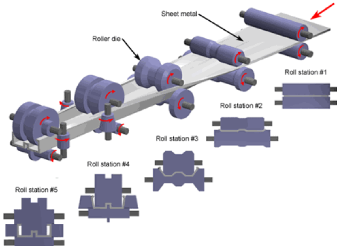
شکل ۲: اشکالی از رول فرمینگ
